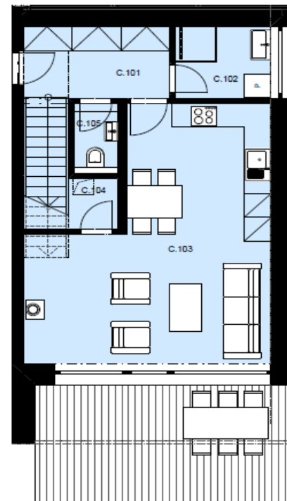
1.NP
